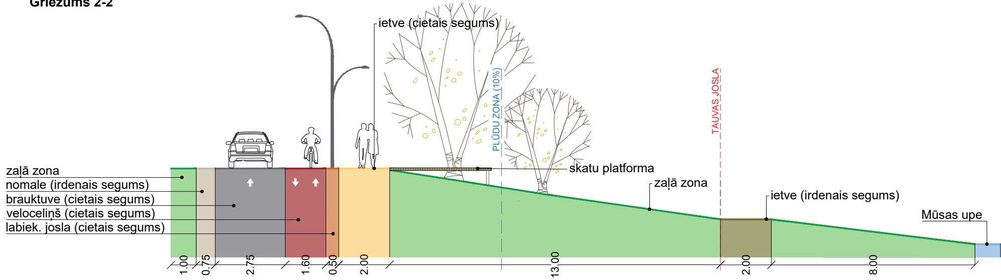
Griezums 2-2
