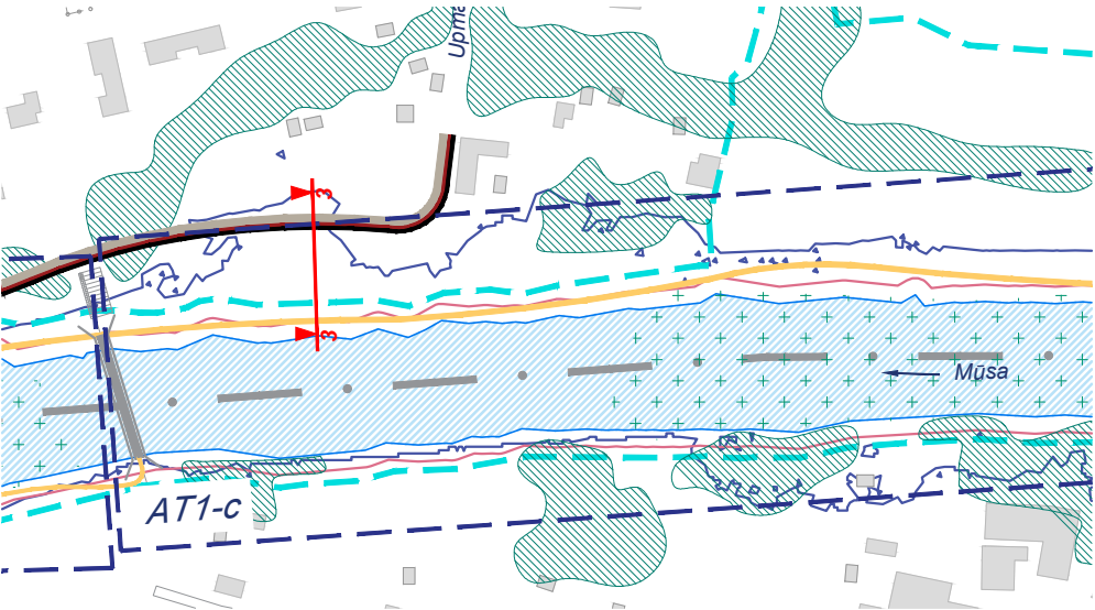
Griezums 3-3, AT1-c Ainavu telpu posmā M 1:5000
